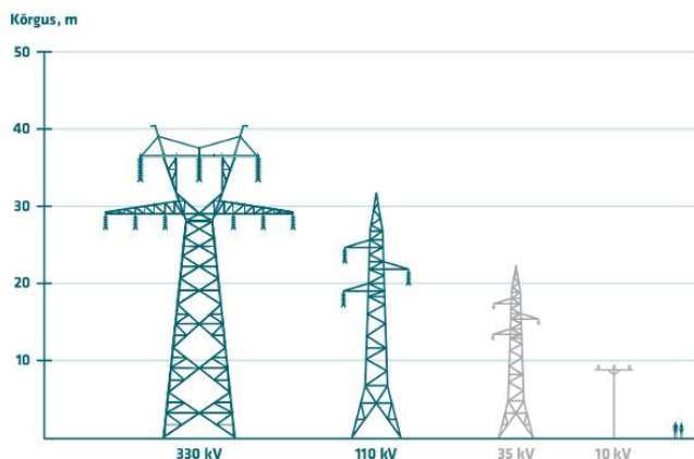
Joonis 57. Erineva pingeklassiga õhuliinide mastid. Allikas: Elering AS
